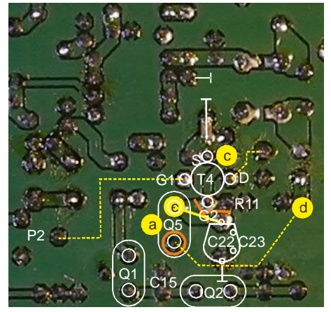
Modifizierte Schaltung
