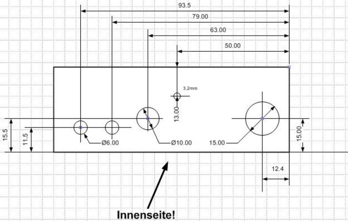
Skizze MA-12 Rückwand - von innen gesehen !
